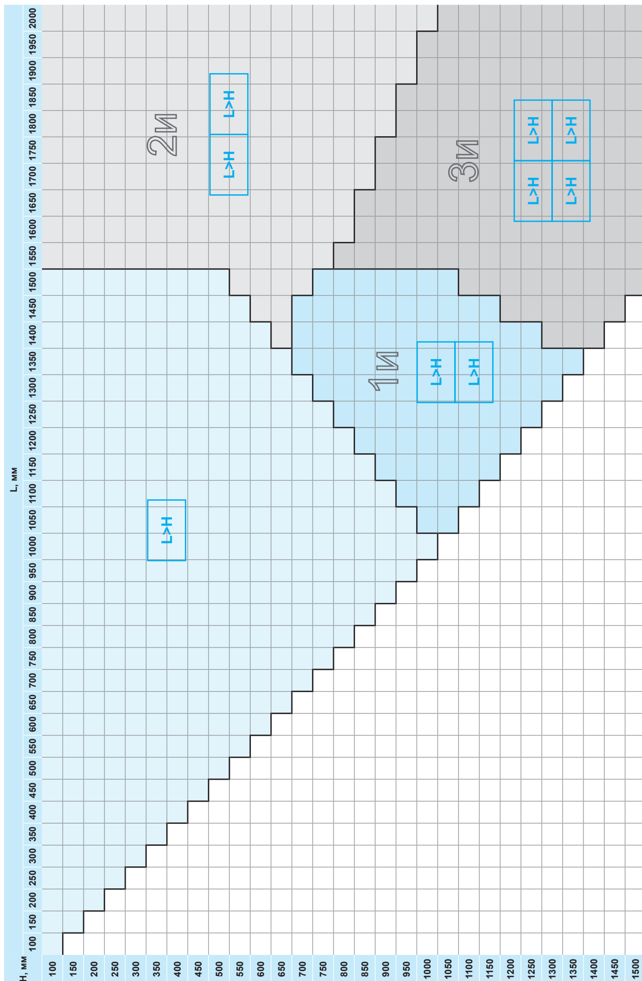
Типоразмеры клапанов ОЗ прямоугольного сечения канального типа
